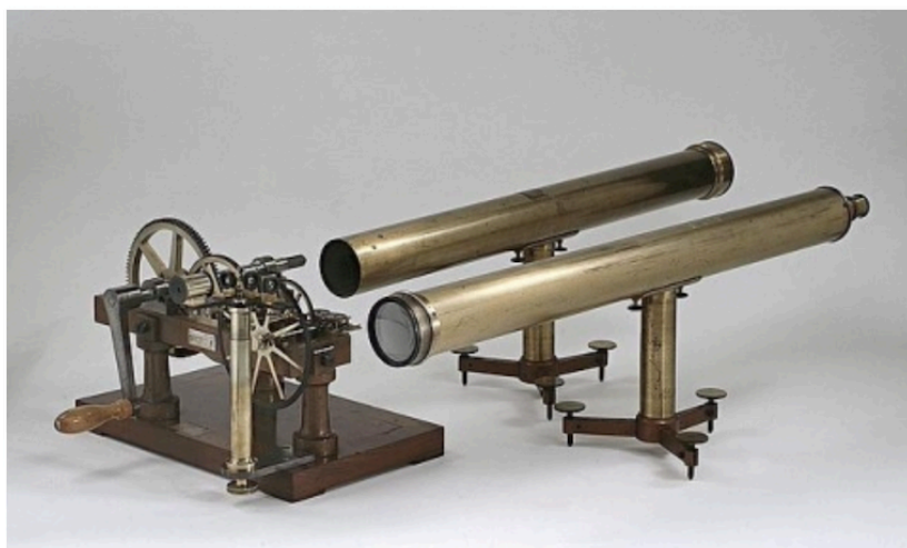
Le dispositif de l'expérience de Fizeau, 1849. Pour reprendre la description qu'en fait Foucault : « M. Fizeau avait placé la lunette à oculaire [à droite de la photo] dans le belvédère d'une maison située à Suresnes, et la lunette à réflexion [au-dessus de la précédente] sur la hauteur de Montmartre, à une distance approximative de 8633 mètres. Le disque [à gauche de la photo], portant sept cent vingt dents, était monté sur un rouage mû par des poids ».
